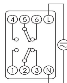
Anschlussdiagramm
