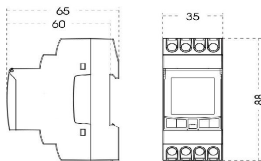
Abmessungen
